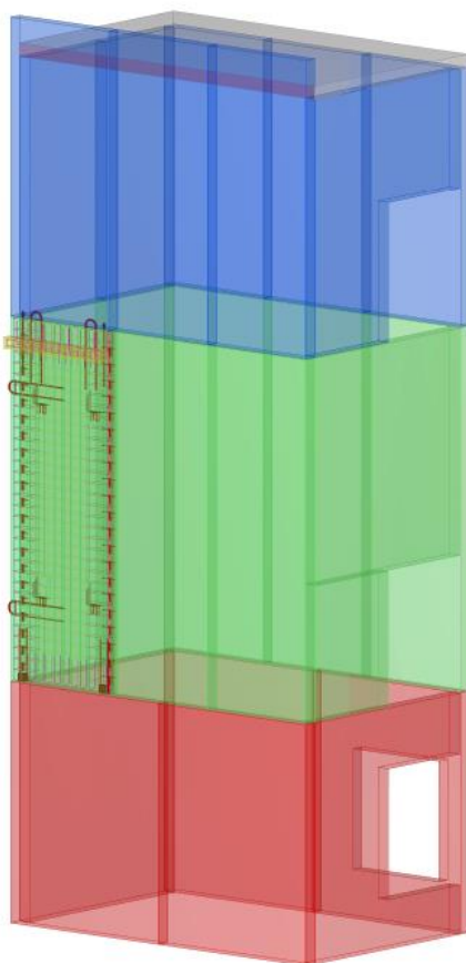
Joonis 4. Trepišahti ja mudeli elemendi täpsus põhiprojekti staadiumis. Joonis: Finnmap Consulting Oy.
