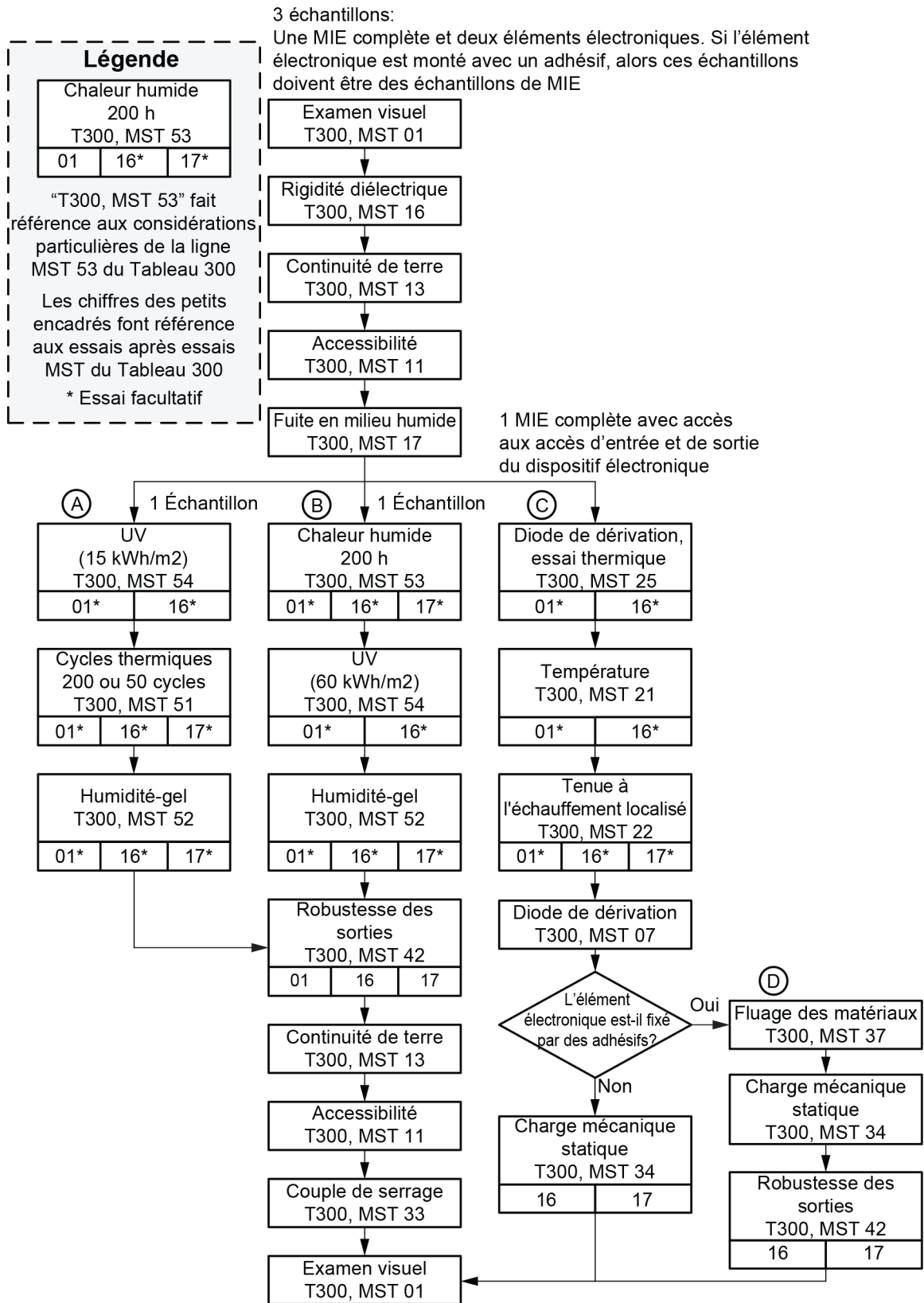
Figure 300 – Séquence d'essais
